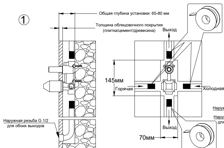
Встраиваемый корпус смесителя без блока
