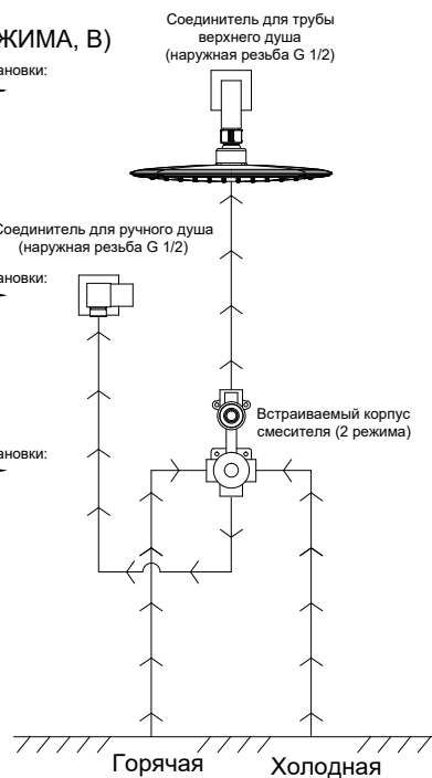
Схема установки водопроводной трубы
