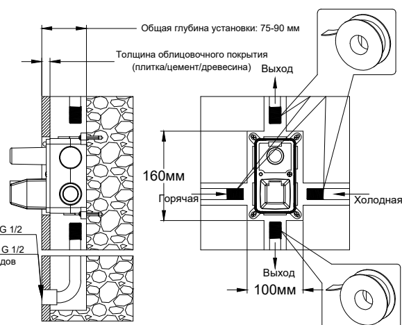
Встраиваемый корпус смесителя с блоком
